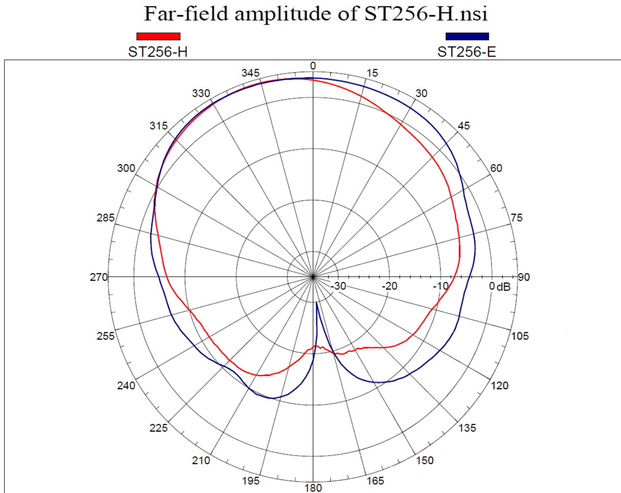
Red Line : H-plane ; Blue Line : E-plane
